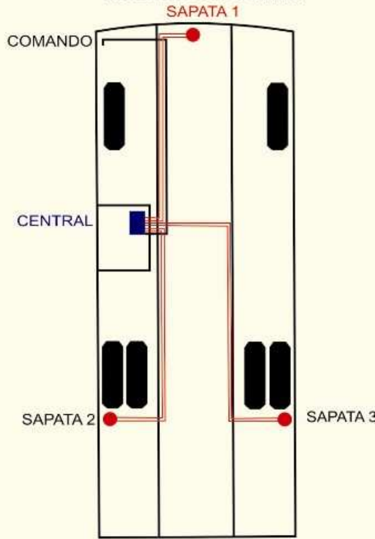
MODELO 3 SAPATAS
